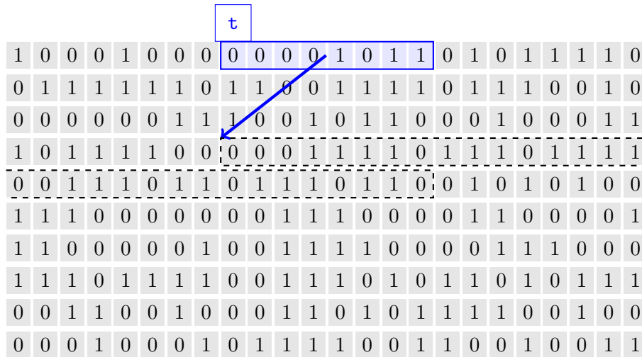
FIGURE 7.2 – Structure en mémoire d'un tableau dynamique déclaré par short int *t = new short int [2]; . Le pointeur t a pour valeur l'adresse 0xB (11 en hexadécimal, 1011 en base 2) de l'espace mémoire alloué à travers la commande new (ici délimité par des pointillés). L'adresse de t est en revanche 0x2 puisque la valeur de t est stockée sur le deuxième octet. L'espace alloué occupe 4 octets, i.e. deux fois la taille d'un short int .
