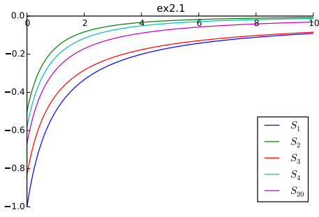
Sommes partielles S_n
