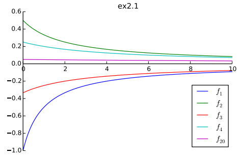
Termes généraux f_n
