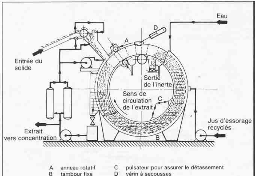
Fig. 15. - Extracteur SATURNE .
