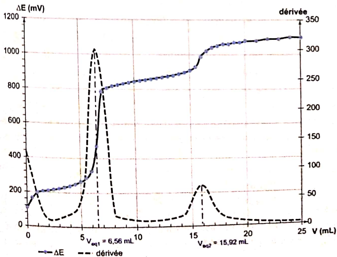
Fig. 2 Dosage d'un mélange d'ions \text{Fe}^{2+} et \text{Co}^{2+} par une solution de sulfate de cérium(IV) avec orthophénanthroline
