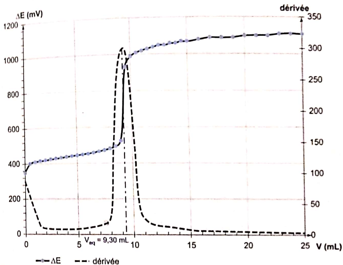
Fig. 1 Dosage d'un mélange d'ions \text{Fe}^{2+} et \text{Co}^{2+} par une solution de sulfate de cérium(IV) sans orthophénanthroline
